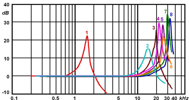
Bild 20: Resonanzfrequenzen typischer Befestigungsarten
