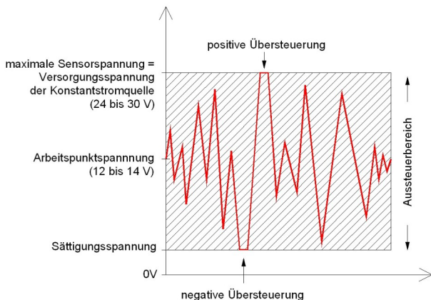
Bild 14: Aussteuerbereich eines IEPE-Aufnehmers
