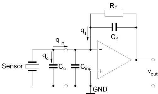
Bild 11: Ladungsverstärker
