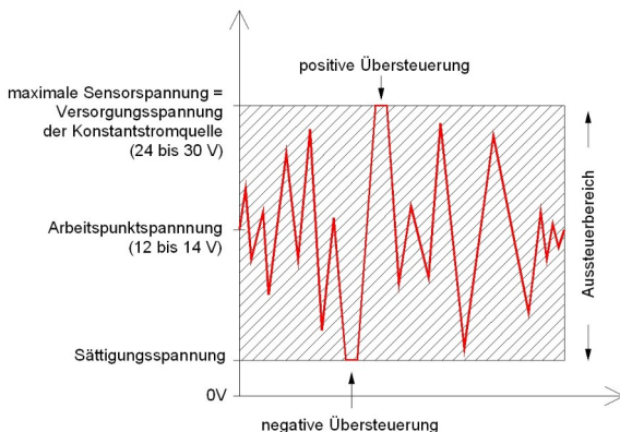
Bild 5: IEPE-Aussteuerergrenzen
