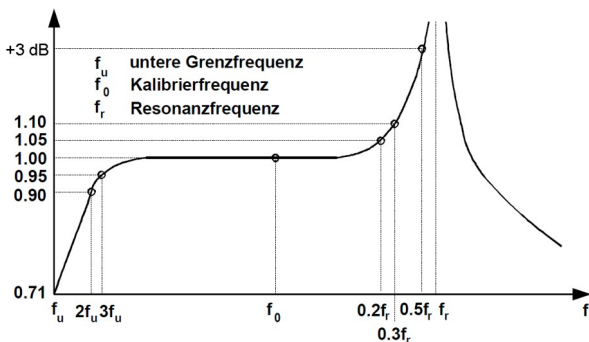
Bild 3: Frequenzgang eines Beschleunigungsaufnehmers
