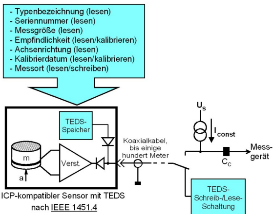
Bild 16: TEDS-Beschleunigungsaufnehmer
