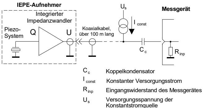
Bild 4: IEPE-Prinzip
