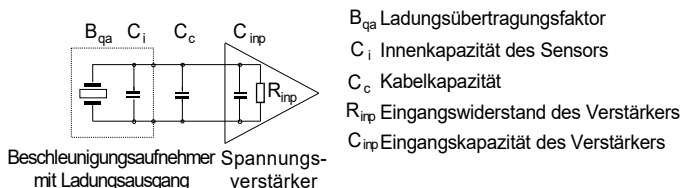
Bild 12: Ladungsaufnehmer an Wechselspannungsverstärker
