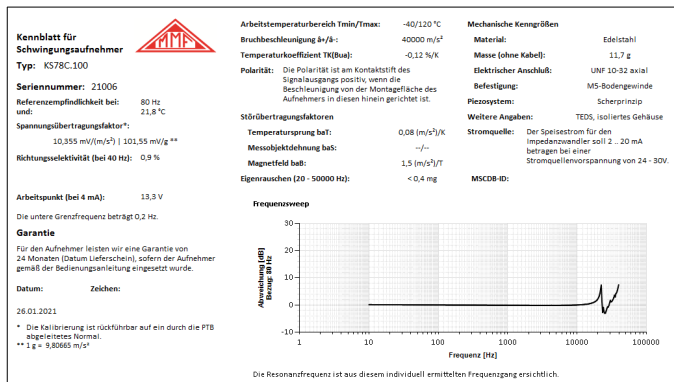
Bild 8: Kennblatt für Metra-Beschleunigungsaufnehmer
