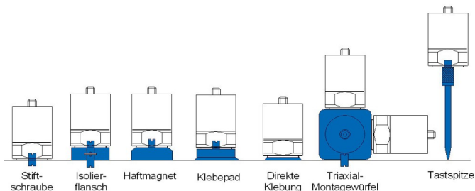
Bild 18: Befestigungsarten für Beschleunigungsaufnehmer
