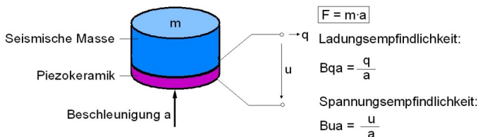
Bild 2: Wirkprinzip eines piezoelektrischen Beschleunigungsaufnehmers
