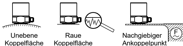
Bild 17: Häufige Ursachen von Ankoppelfehlern
