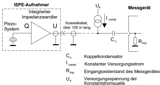
Bild 13: IEPE-Prinzip
