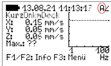
Bild 19: AskSensors-Indikator
