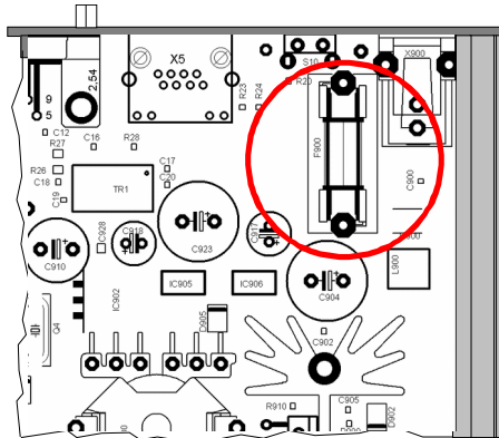
Bild 8: Sicherungshalter
