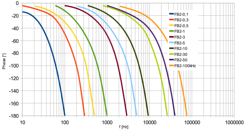
Bild 30: Phasenfrequenzgang des M208A mit den Tiefpassfiltern FB2-...
