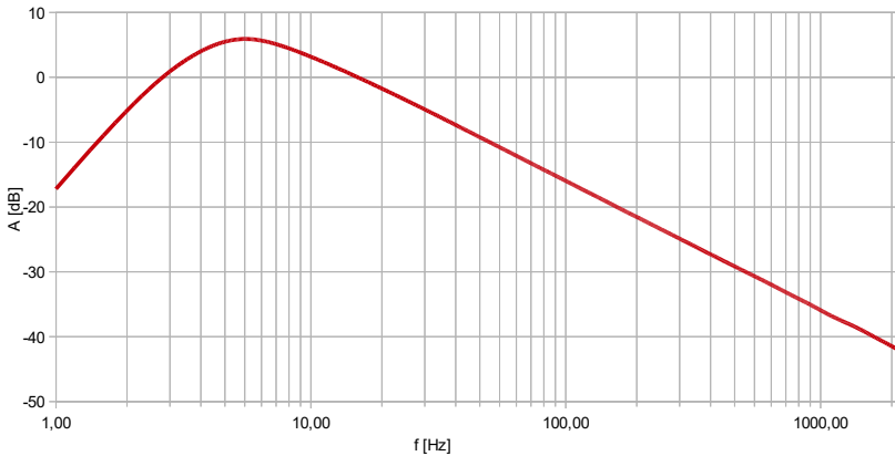
Bild 31: Amplitudenfrequenzgang des M208A mit dem Einfachintegrator FBV
