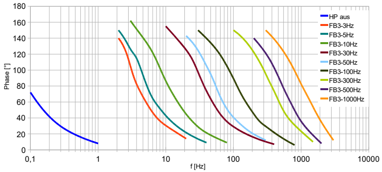
Bild 28: Phasenfrequenzgang des M208A mit den Hochpassfiltern FB3-...
