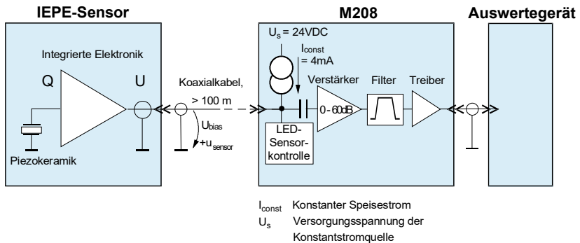
Bild 3: IEPE-Prinzip
