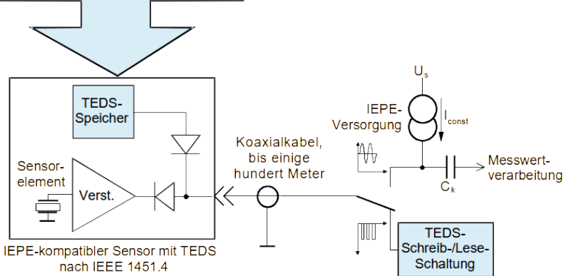
Bild 5: TEDS-Prinzip
