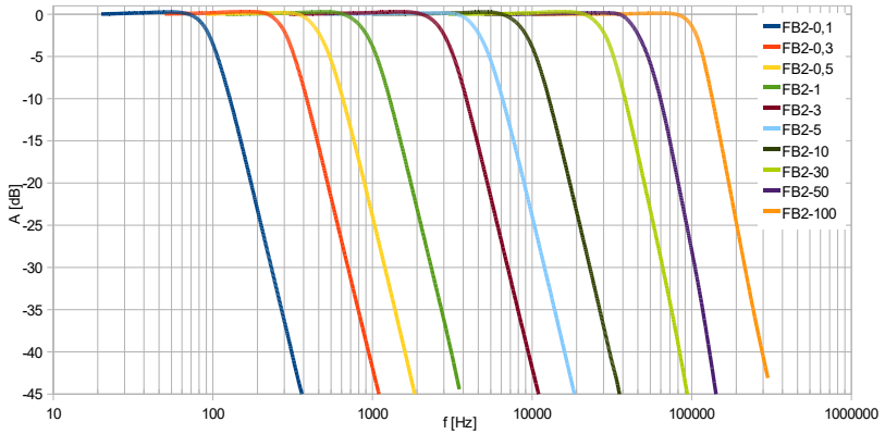
Bild 29: Amplitudenfrequenzgang des M208A mit den Tiefpassfiltern FB2-...
