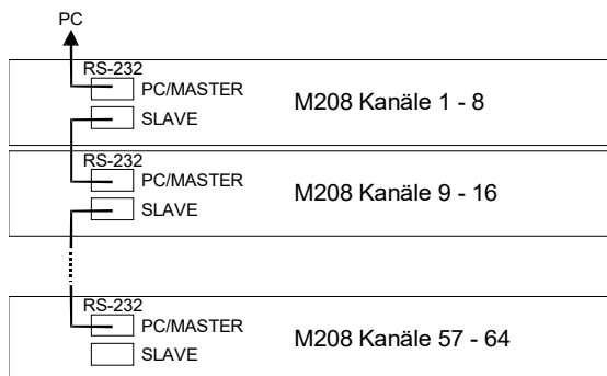
Bild 42: Vernetzung mehrere Geräte über die seriellen Schnittstellen
