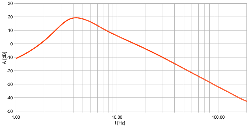
Bild 32: Amplitudenfrequenzgang des M208A mit dem Doppelintegrator FBD
