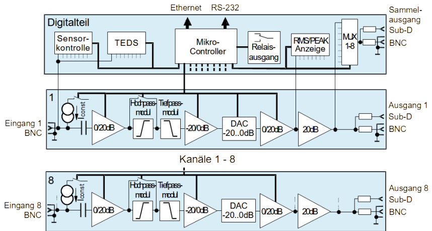
Bild 6: Blockschaltbild
