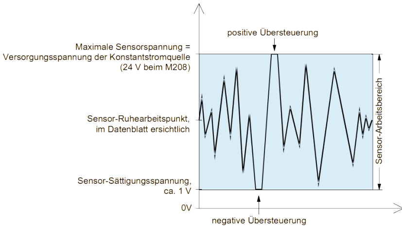
Bild 4: Sensor-Aussteuergrenzen
