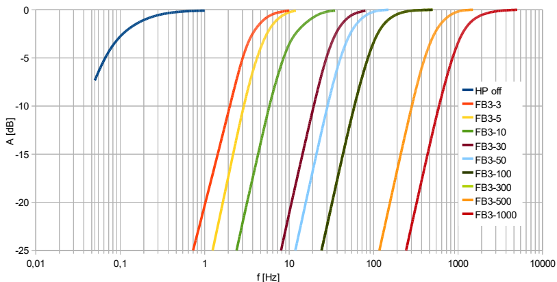
Bild 27: Amplitudenfrequenzgang des M208A mit den Hochpassfiltern FB3-...
