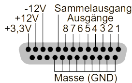
Bild 10: Anschlussbelegung der Sub-D-Buchse auf der Rückseite
