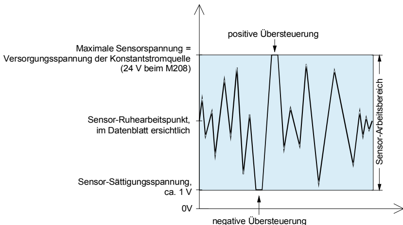
Bild 3: Sensor-Aussteuerergrenzen
